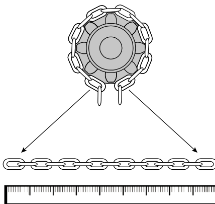
CIRCONFERENZA BARBOTIN
