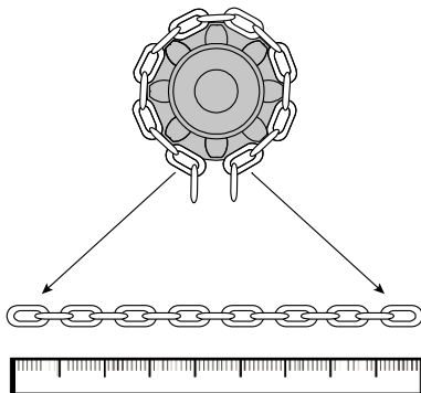
CIRCONFERENZA BARBOTIN
